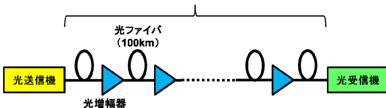
図1 伝送実験系構成
